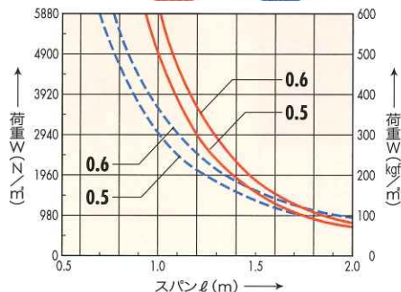
単純梁
