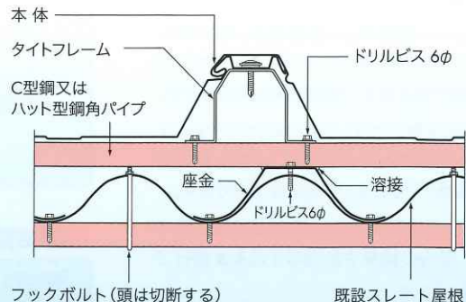
●スレート屋根 改修断面図
