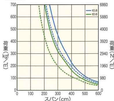
連続梁
