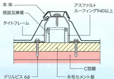
●瓦棒葺 改修断面図（鉄骨下地）
