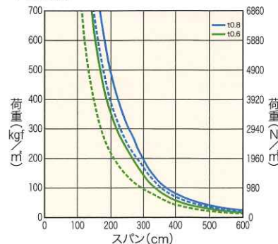
片持ち梁
