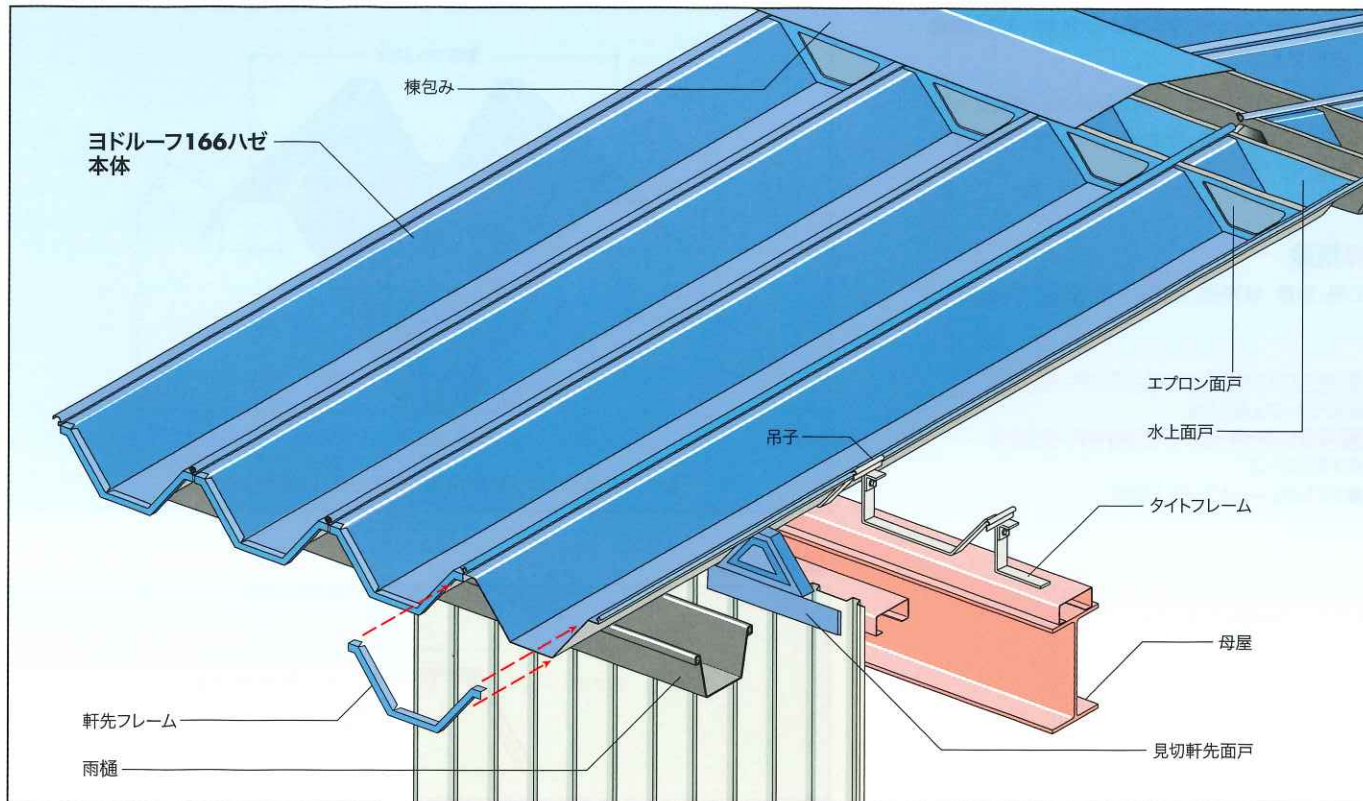
■ヨドルーフ166ハゼ 構成図
